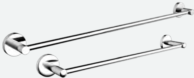
EST03/EST06 - SINGLE TOWEL RAIL EST03 W - 495 D - 55 P - 85 C - 440 EST06 W - 638 D - 50 P - 56 C - 588
